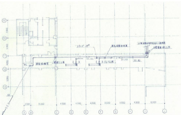
クリーンセンター 3F ⑨-⑬間 平面図 S=1/200
