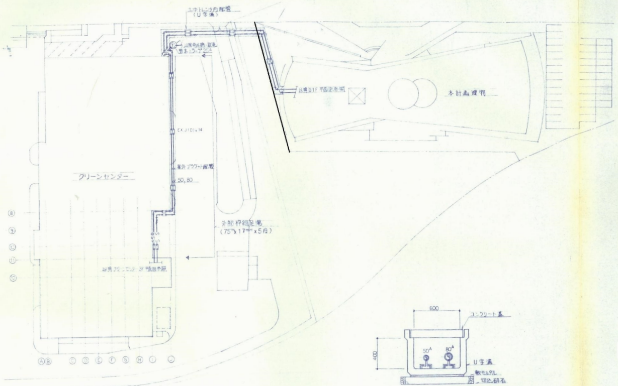
トレンチ内配管断面図 S=1/20
