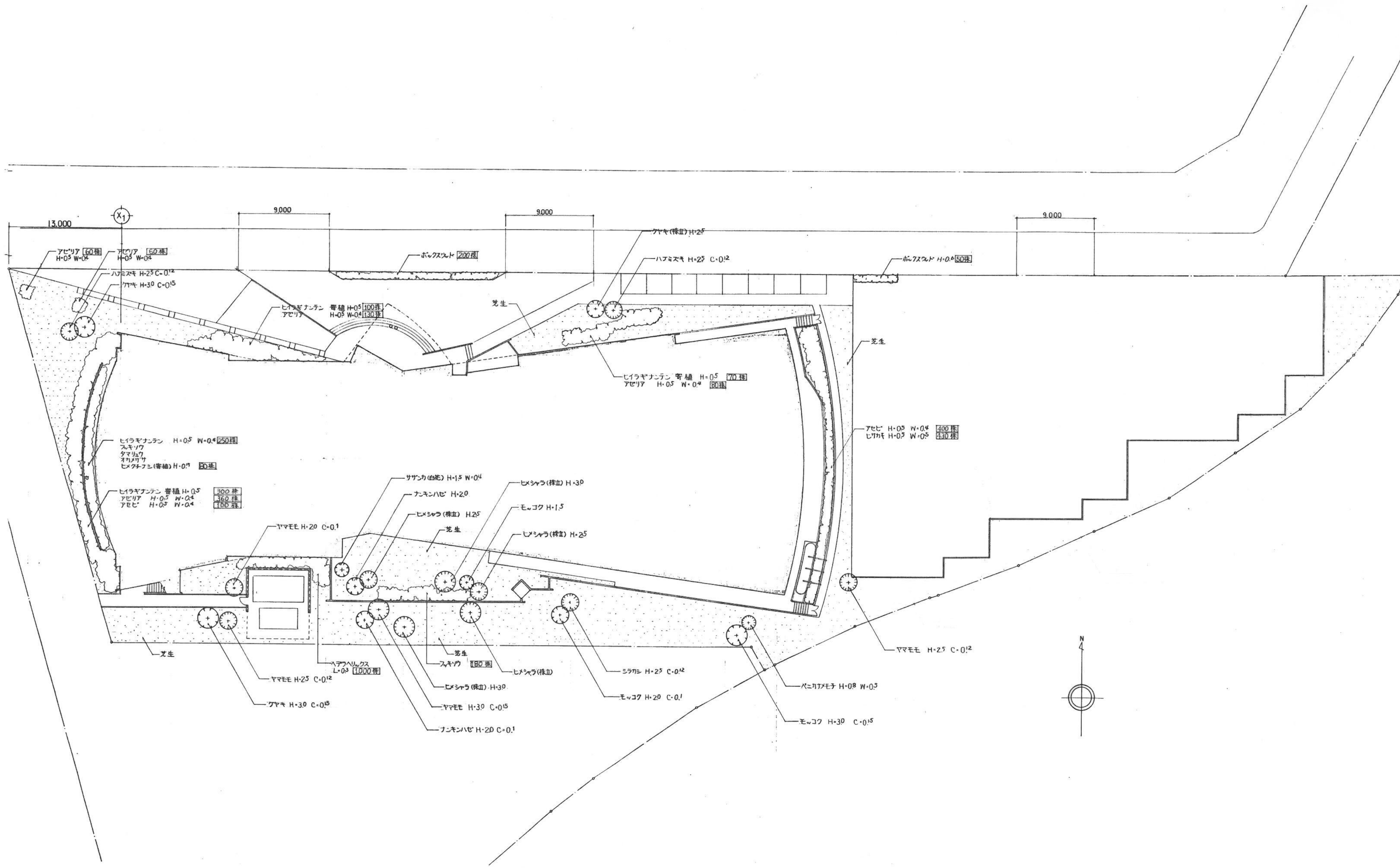
植栽図
