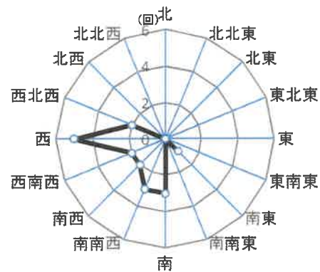
風向の出現頻度(29回計測中)
