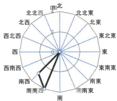
図 3-3 風向の出現頻度（千葉県データ）
